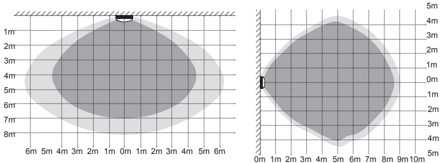
Установка на потолок
